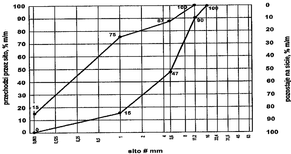
Rys. 2. Krzywe graniczne uziarnienia mieszanki kruszyw 0/11,2 mm do górnej warstwy podłoża ulepszono
