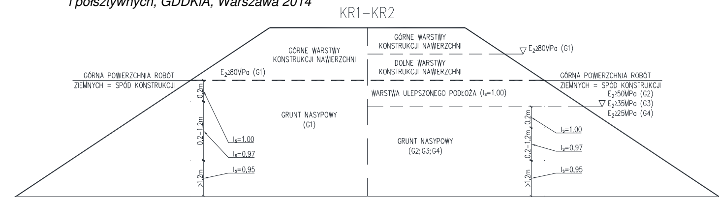
Rysunek 1: Schemat układu warstw konstrukcji nawierzchni dla kategorii ruchu KR1-KR2 w nasypie oraz wymagane wartości wtórnych modułów odkształcenia na powierzchni warstw w przypadku grupy nośności podłoża G1 oraz w przypadku grupy nośności podłoża G2, G3 i G4 – opracowano na podstawie: Katalog typowych konstrukcji nawierzchni podatnych i półsztywnych, GDDKiA, Warszawa 2014
