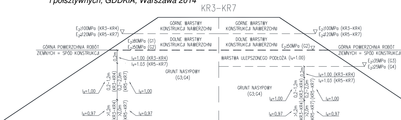
Rysunek 2: Schemat układu warstw konstrukcji nawierzchni dla kategorii ruchu KR3-KR7 w nasypie, oraz wymagane wartości wtórnych modułów odkształcenia na powierzchni warstw w przypadku grupy nośności podłoża G1 i G2, oraz w przypadku grupy nośności podłoża G3 i G4 – opracowano na podstawie: Katalog typowych konstrukcji nawierzchni podatnych i półsztywnych, GDDKiA, Warszawa 2014
